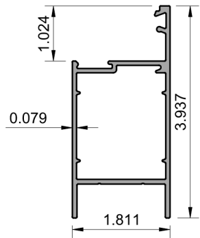
6 TOP & BOTTOM RAIL YYS048 6063-T5
