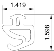
12 EPDM GASKET SBW-26955
