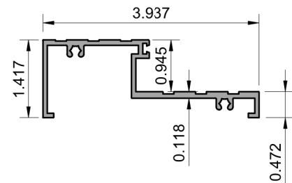
17 DOOR SILL SPA10049 6063-T5
