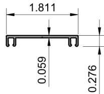
9 DOOR RAIL ADAPTOR SPA10108 6063-T5
