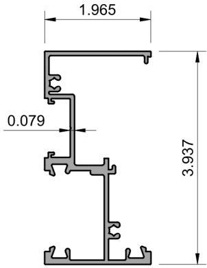
1 DOOR FRAME SPA10001 6063-T5
