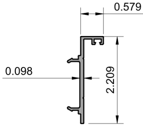
2 DOOR ADAPTOR SPA10013 6063-T5
