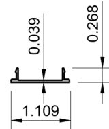
5 DOOR ADAPTOR SPA 13006 6063-T5
